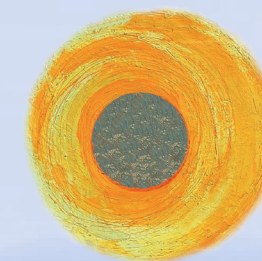
Strahlenkranz bei Sonnenfinsternis
